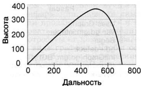
Рис. КП.2 Движение тела под углом 45^\circ с начальной скоростью 600 \text{ м/с}
