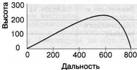
Рис. КП.3 Движение тела под углом 30^\circ с начальной скоростью 600 \text{ м/с}
