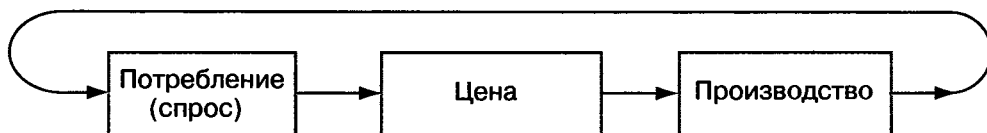
Рис. 5.11 Простейшая экономическая модель
