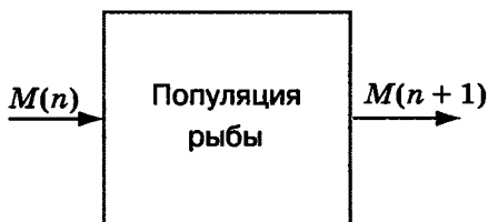
Рис. 5.3 Модель изменения возобновляемого ресурса
